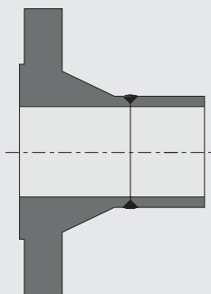
Bride à souder à collerette
