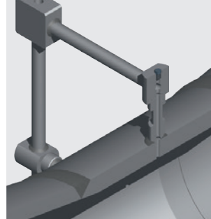
Prises de pression à chambre annulaire réalisée en tubes
