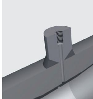
Prise NPT / embout à souder
