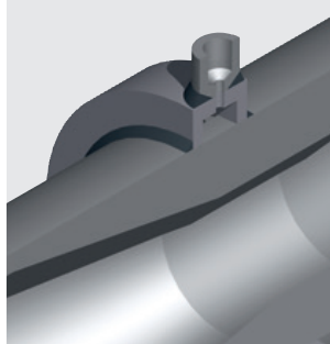
Prises de pression à chambre annulaire réalisée par bague soudée
